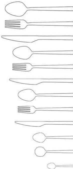
Yemek Kaşık / Table Spoon / 304 18-10 3 mm / 42,5 mm / 11,5 mm / 206 mm / 53 gr
